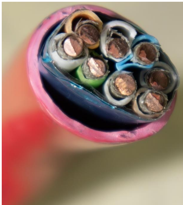
Ryc. 4. Przekrój kabla HTKSHekw PH120/FE180/E30-E90 4x2x2,8
