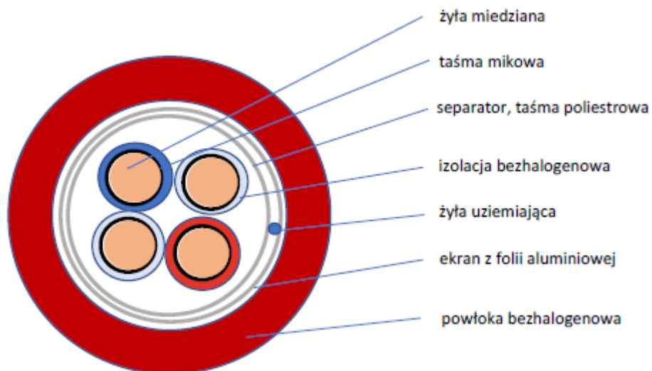
Ryc. 2. Przekrój kabla HTKSHekw PH120/FE180/E30-E90
