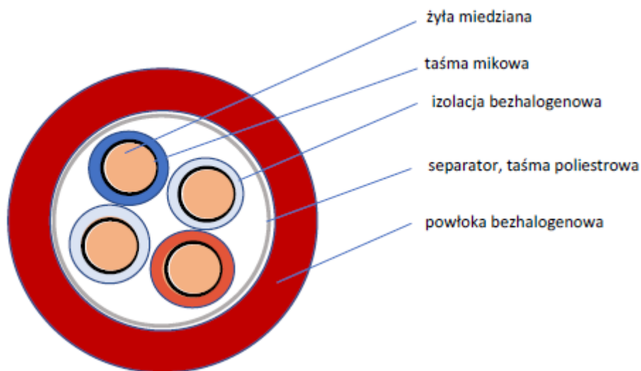
Ryc. 1. Przekrój kabla HTKSH PH120/FE180/E30-E90
