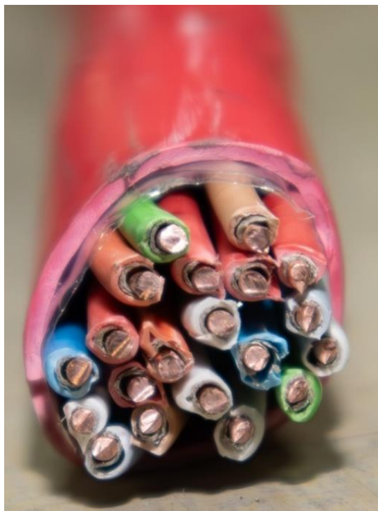
Ryc. 2. Przekrój kabla HTKSH PH120/FE180/E30-E90 10x2x1,8
